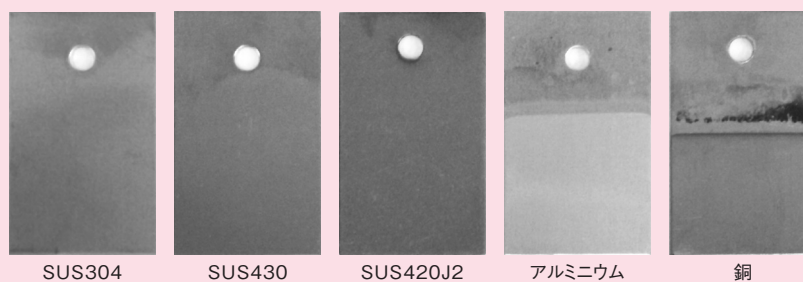
図1 サラサイドに金属テストピースを浸漬した場合の変化
